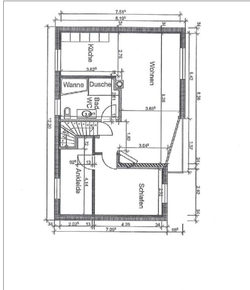
Dachgeschoss
